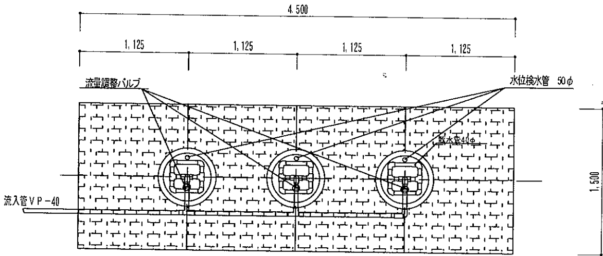
PPP-21~30人槽 平面図
