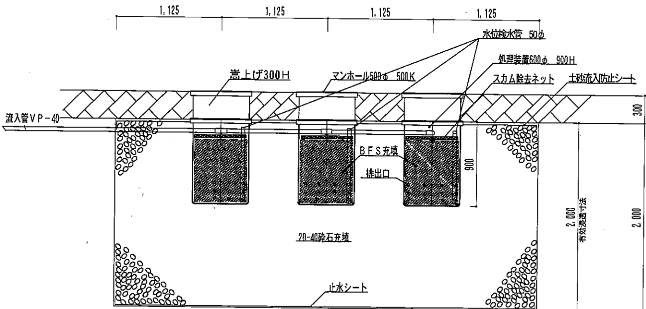
PPP-21~30人槽 断面図
