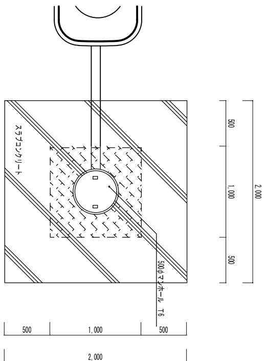
駐車場仕様平面図 S 1:30
